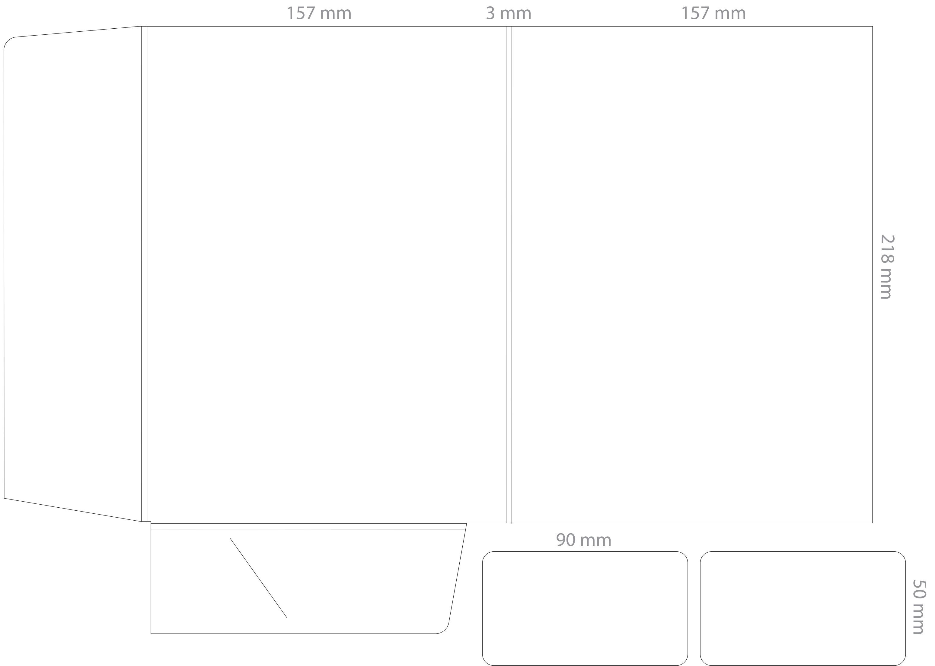
Výseková forma S07
