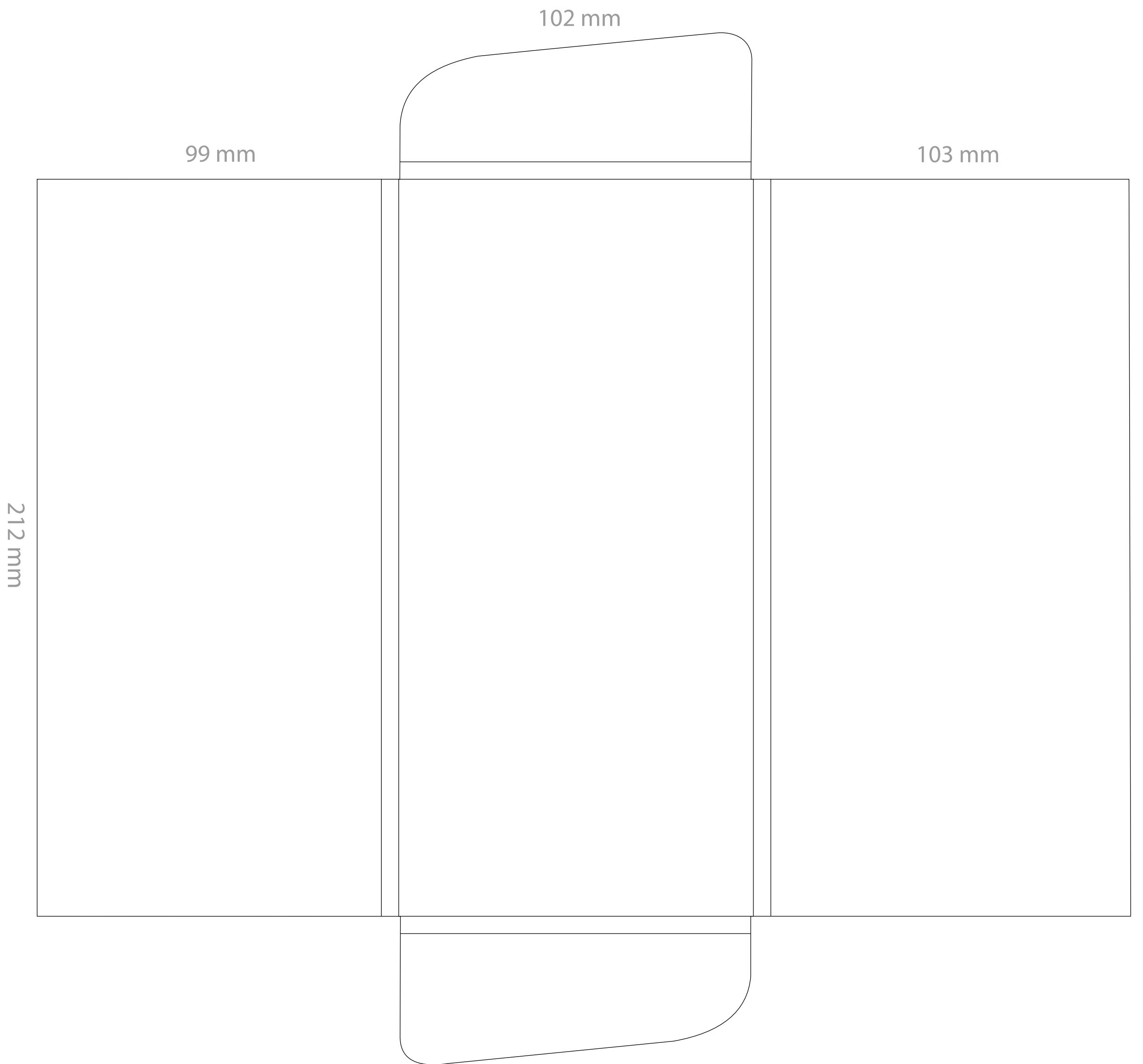
Výseková forma S24
